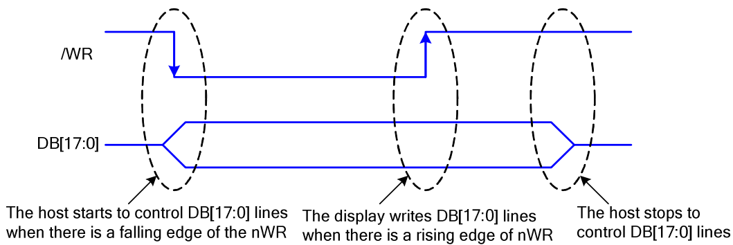
Fig. 9.2 8080-Series /WR Protocol
